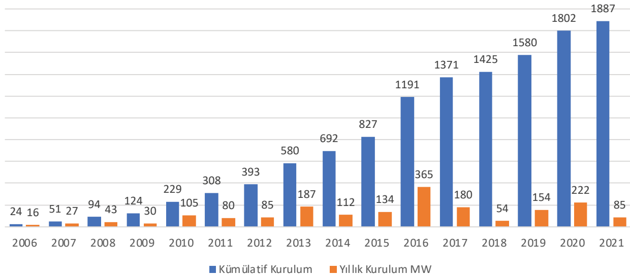
ŞEKİL 8.2. İzmir Bölgesi Rüzgâr Enerjisi Kurulu Güç (MW) (2006-2021, TÜREB)
