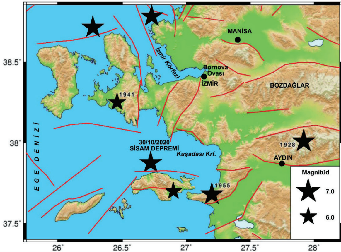
ŞEKİL 9.2. İzmir ve Çevresinde Meydana Gelmiş Önemli Depremler ve Fay Hatları
