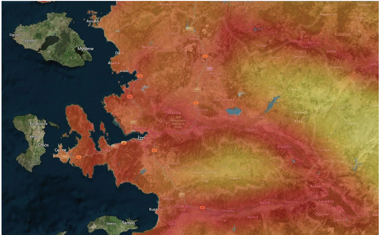
ŞEKİL 9.1. AFAD Deprem Tehlike Haritası
