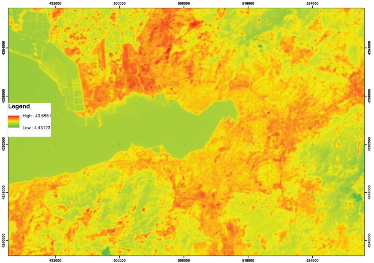
ŞEKİL 8.9. İzmir Bölgesi'nde Yüzey Sıcaklıkları
