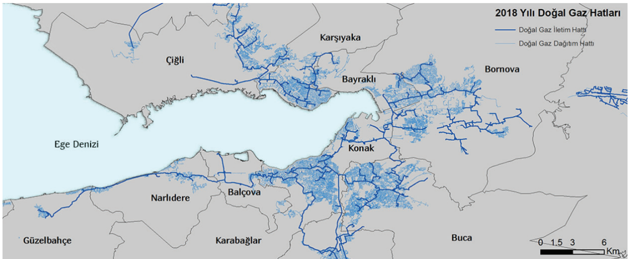
ŞEKİL 6.20. İzmir Bölgesi Doğal Gaz Ağı
